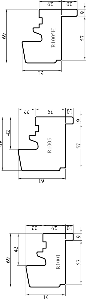
Appui rénovation
