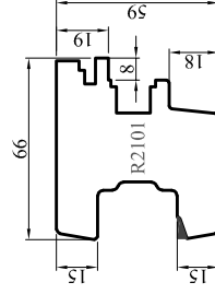
Battement central
